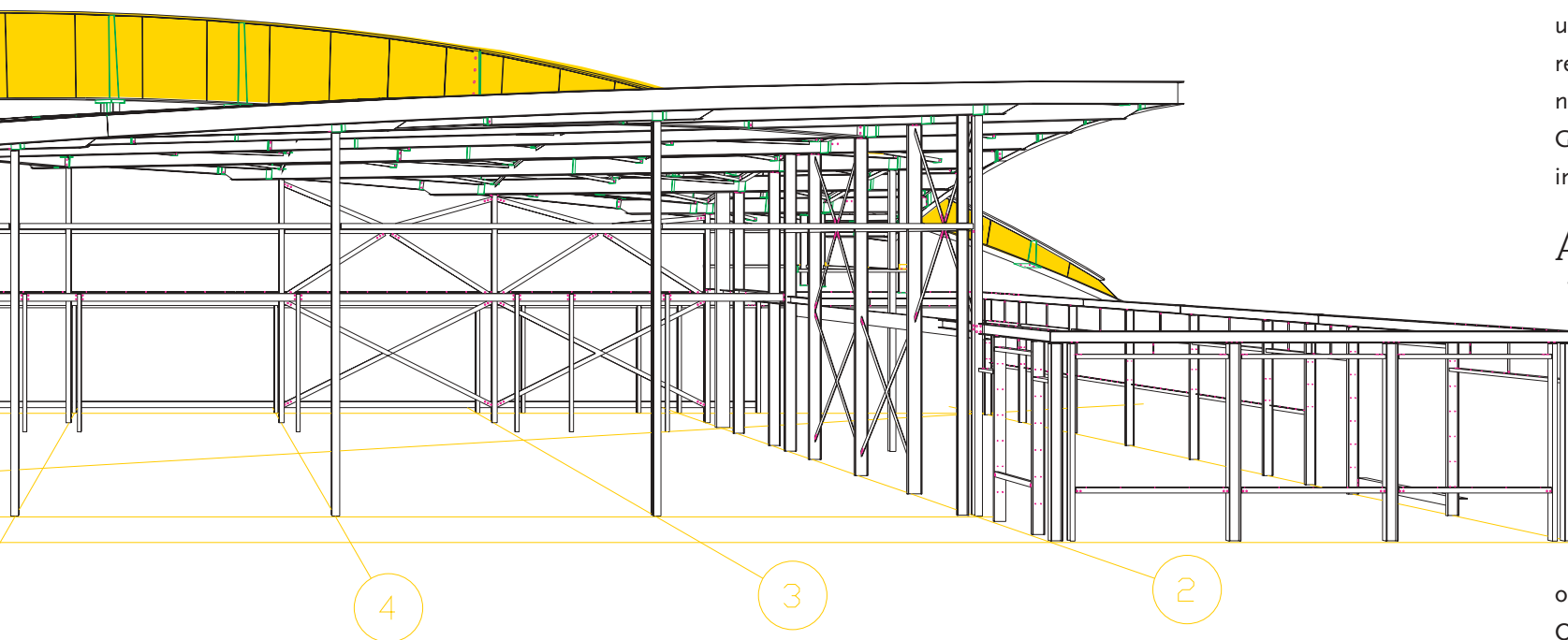
Staalconstructietekening Brandweerpost Vijfhuizen
